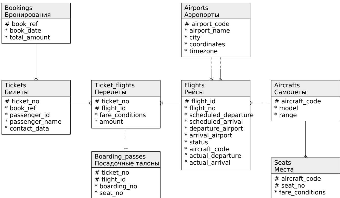
Рисунок М.2. Диаграмма схемы Bookings
