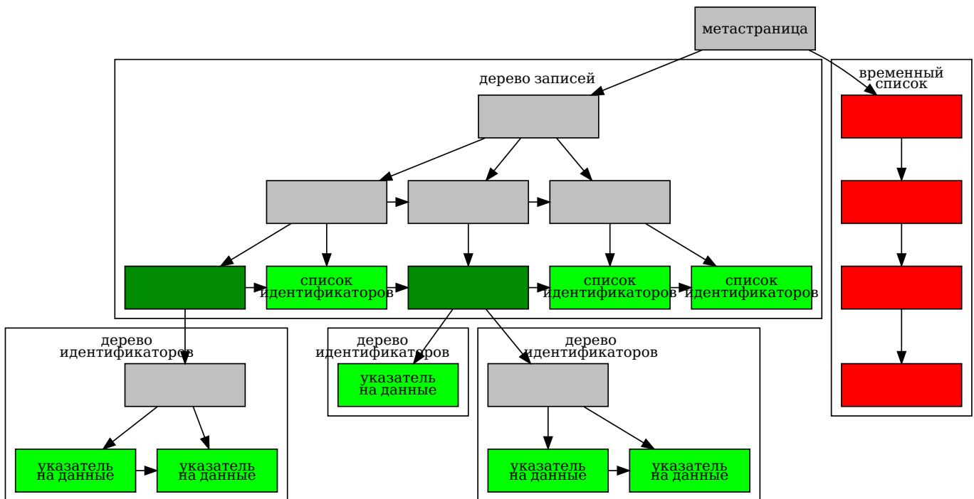
Рисунок 62.1. Внутреннее устройство GIN
